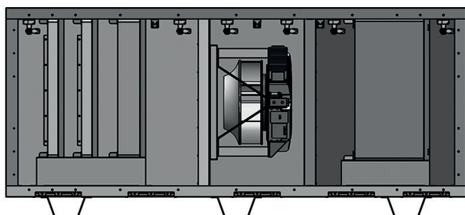
C. Filtro Metálico / Merv 8 / Merv 13 / Luz UV / HEPA 99.99%
