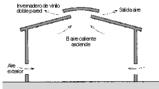
Figura 1. Ventilación natural
