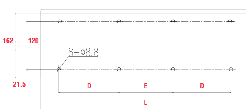
Modelo 36/48 tamaño de la placa de montaje
