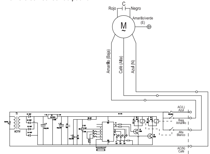
3) Diagrama esquemático de cableado del control remoto con sensor de puerta
