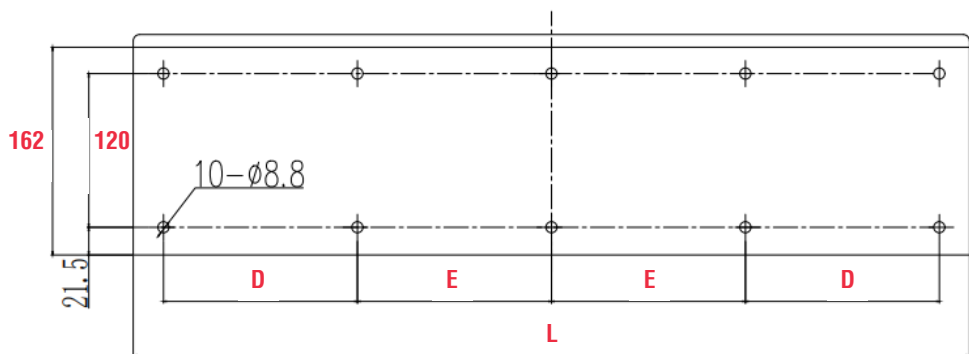
Modelo 60 tamaño de la placa de montaje
